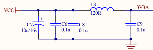
电源引脚附近放置0.1uF旁路电容,减少电源噪声
