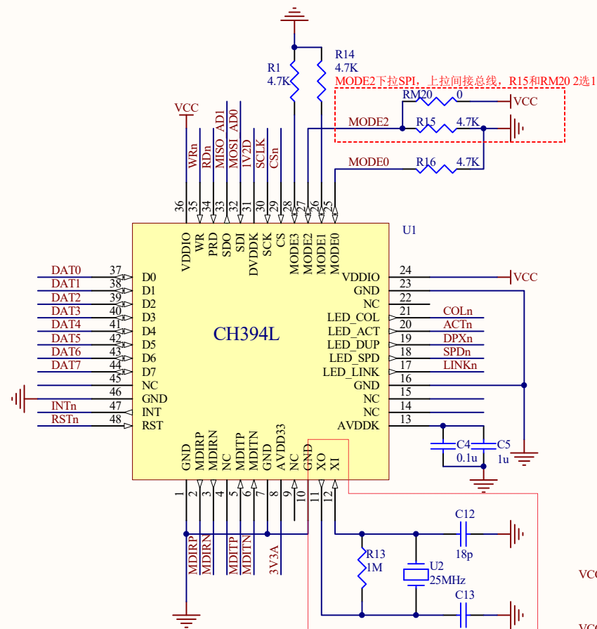
11,12 脚及器件分别远离干扰,晶体靠近芯片
