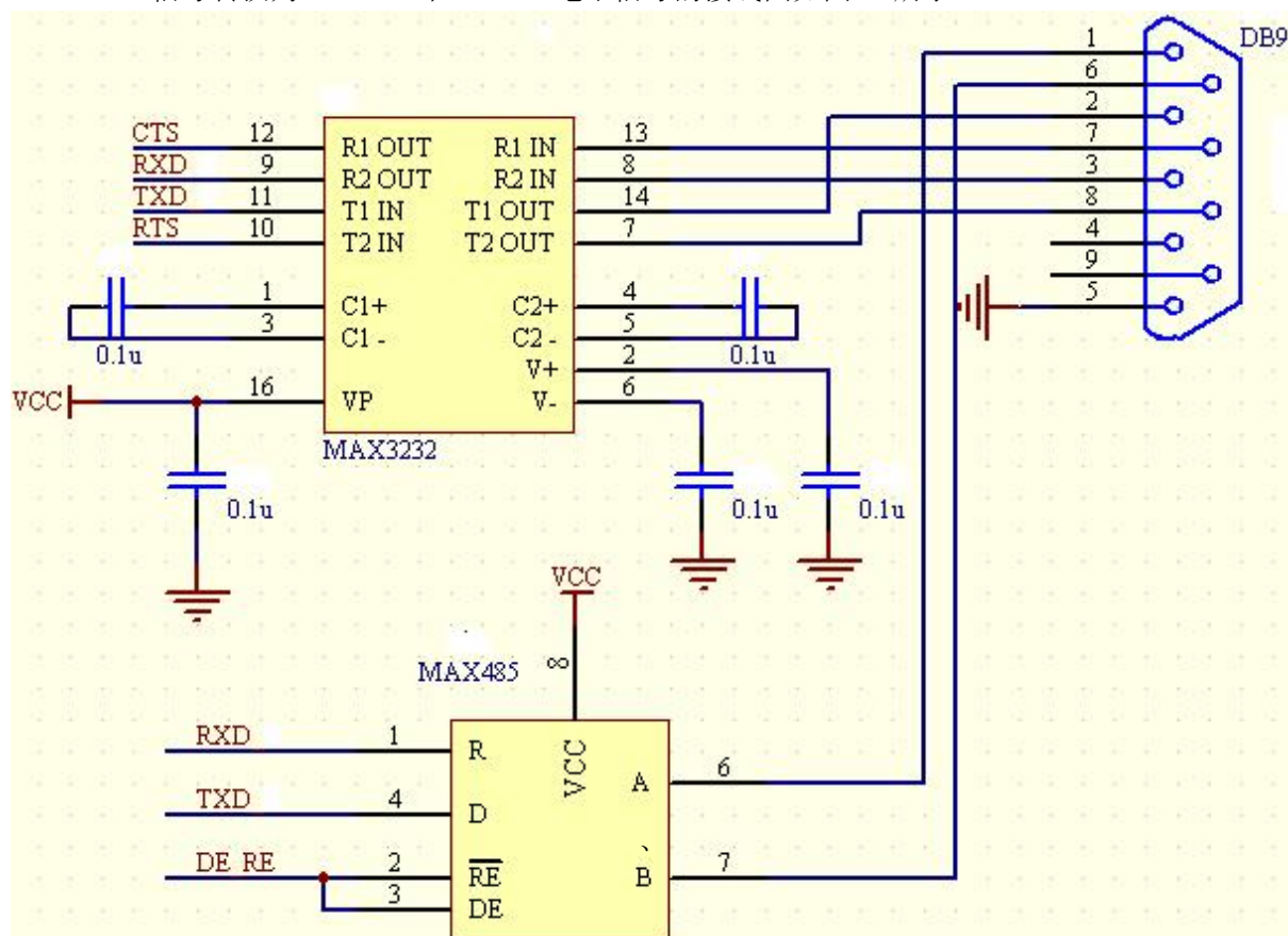
图2.5 UART信号转换为RS-232C或RS-485的接线图
