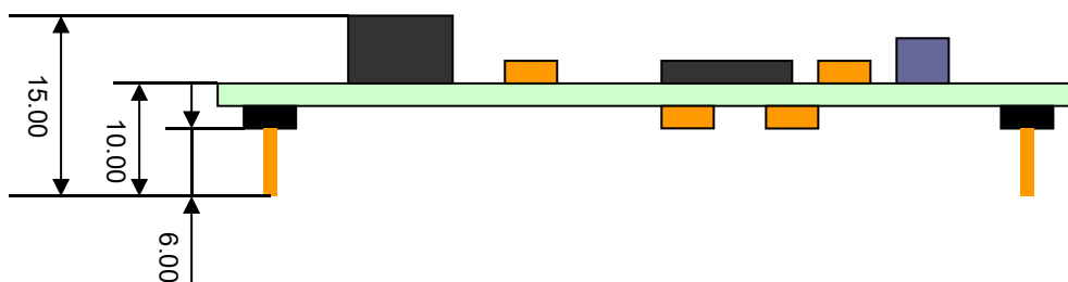
图2.1 SKT-LAN-010尺寸图
