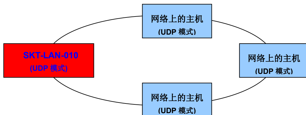
图 4.7 SKT-LAN-010 工作在 UDP 模式的逻辑图
