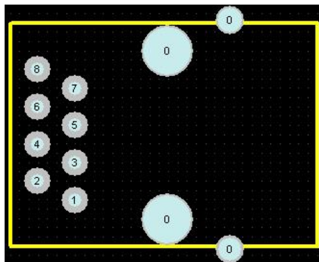
图2.4为RJ-45的PCB引脚定义图
