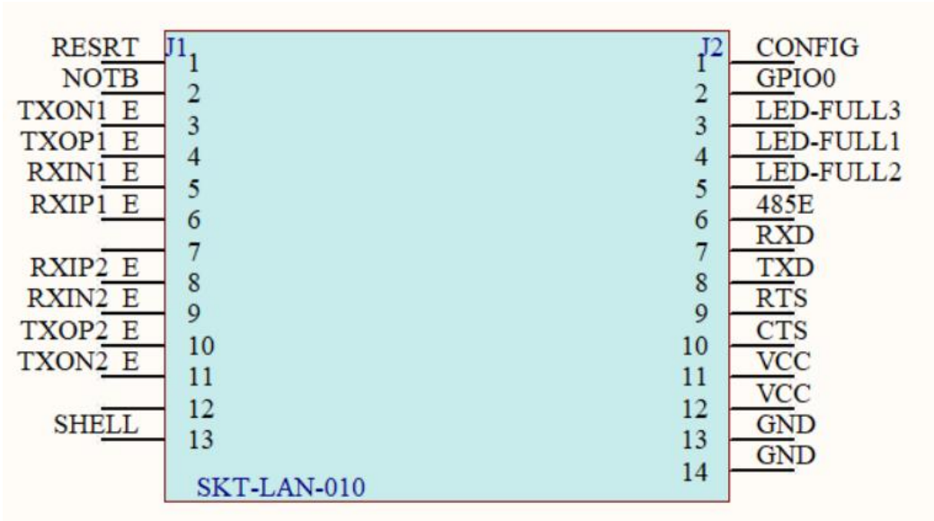
图2.2 SKT-LAN-010引脚排列示意图
