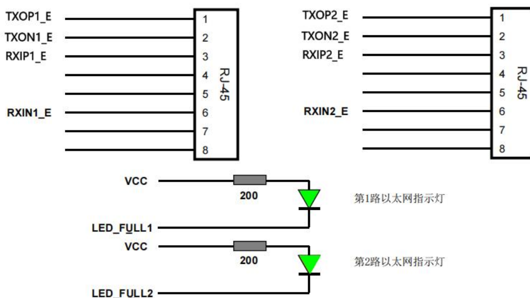
图2.3 SKT-LAN-010与RJ-45的连接
