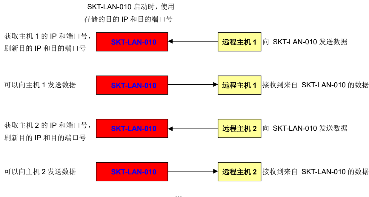
图 4.8 ATSR=2 时 SKT-LAN-010 自动刷新目的 IP 和目的端口号
