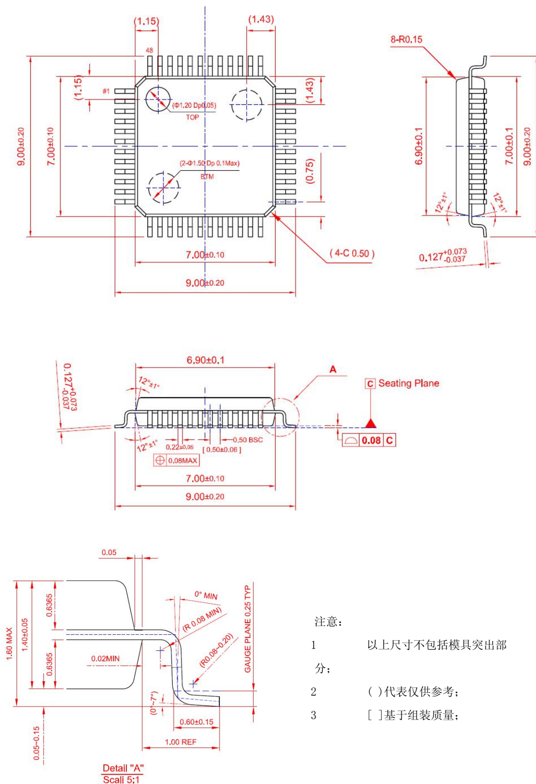
图 25 封装描述
