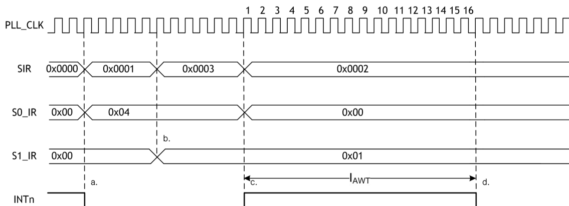
图 21 INTLEVEL 时序
