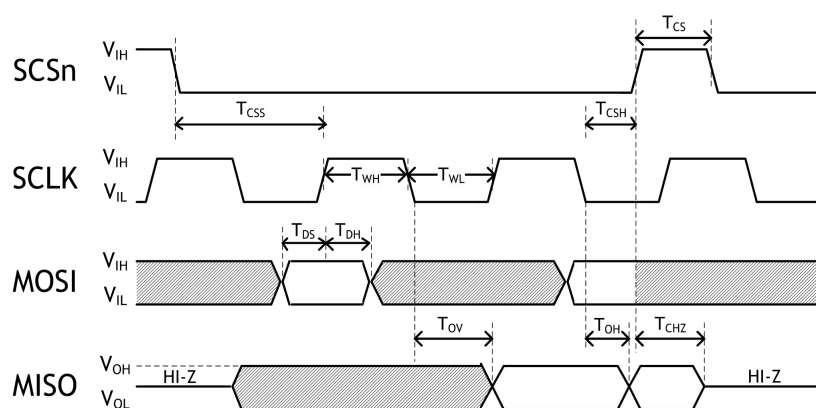
图 23 SPI 时钟
