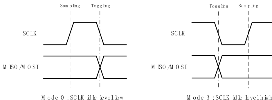
图 6 SPI 模式 0 和 3
